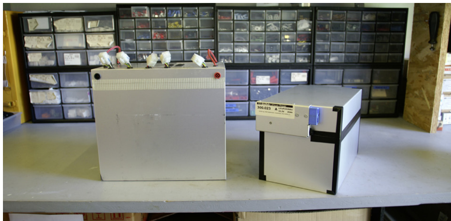
Die Batteriezellen aus dem ausgebauten Batteriepack eines Twikes (links) werden geprüft und dann in 2nd-Life-Speichermodule (rechts) eingebaut. (Bilder: B. Vogel)
