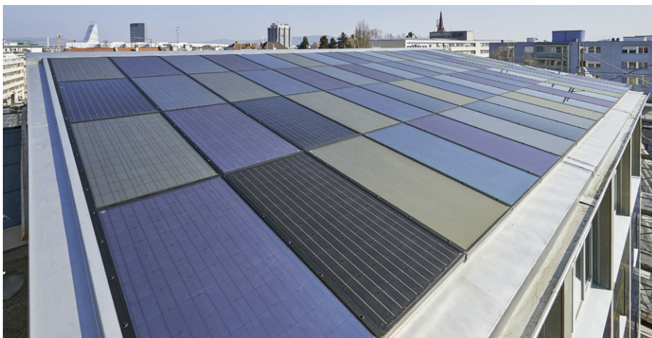
Das ehemalige Kohlesilo im Gundeldinger Feld in Basel: PV-Zellen in Grün, Gold, Blau und Grau liefern bis zu 20 kW p . Der Strom wird seit Herbst 2015 in einem 2nd-Life-Batteriespeicher gepuffert. (Bilder: Martin Zeller)
